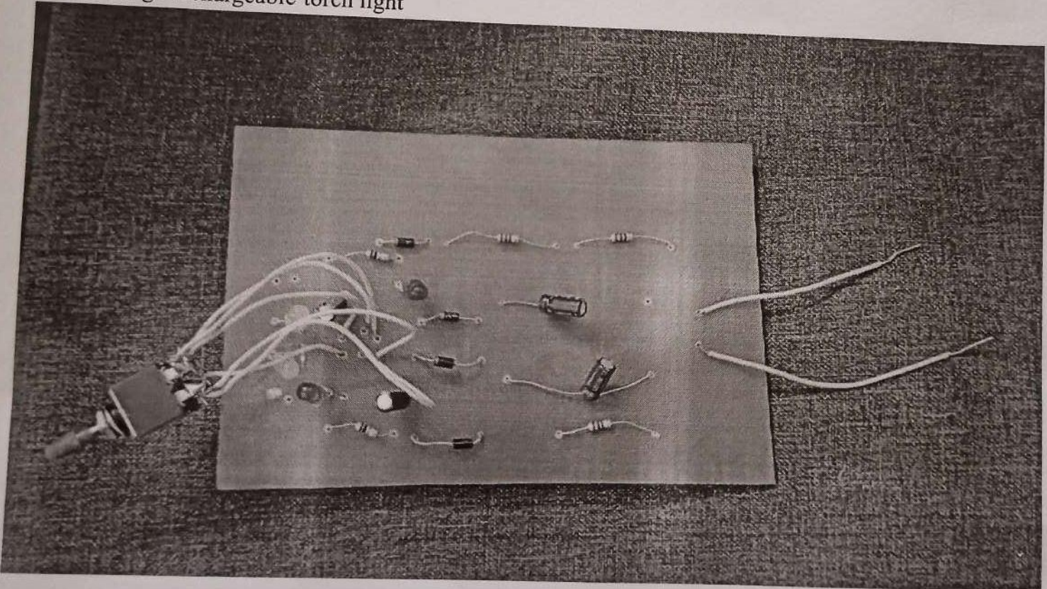
IR Remote tester
